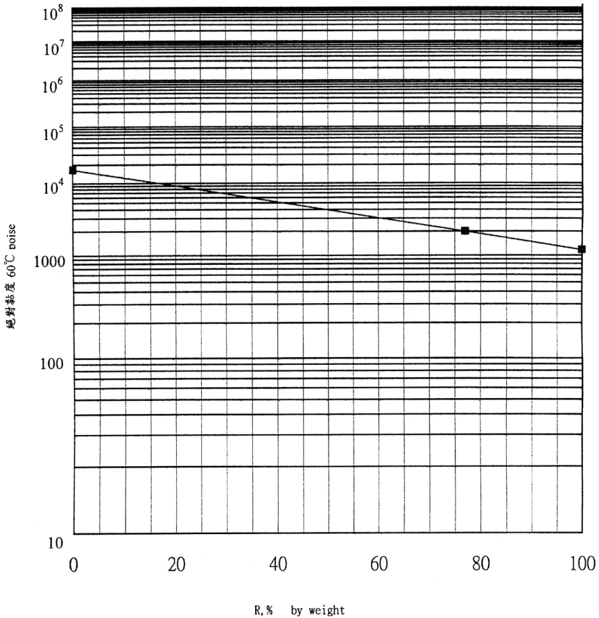
圖 5.1 RAP黏滯度與R關係圖
